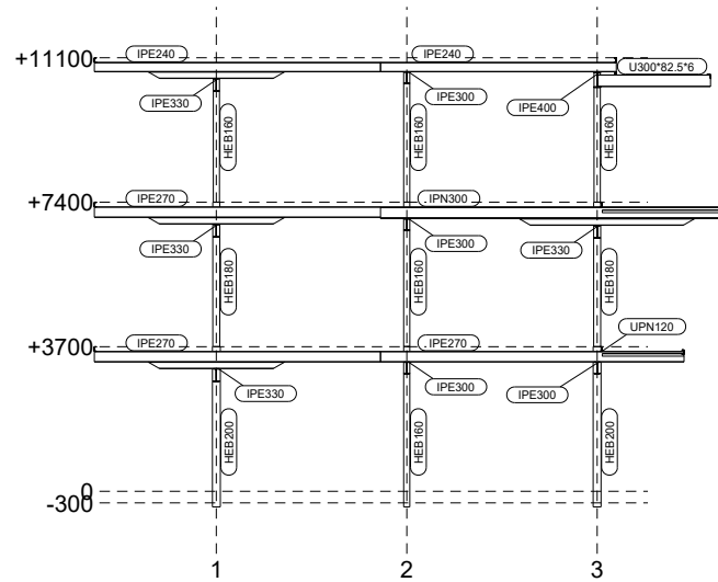
Sección A - A 1:150
