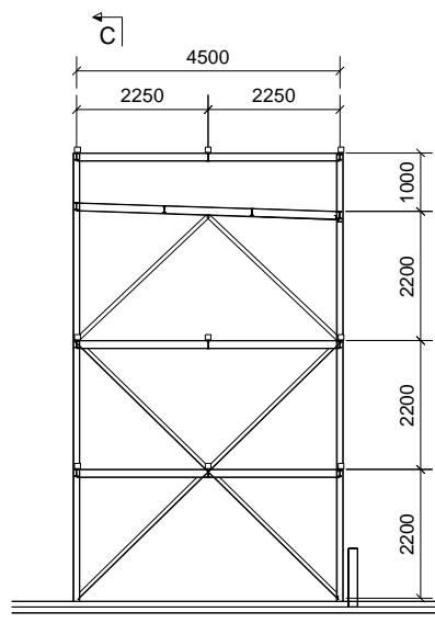
Sección A - A 1:100
