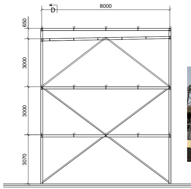
Sección B - B 1:100
